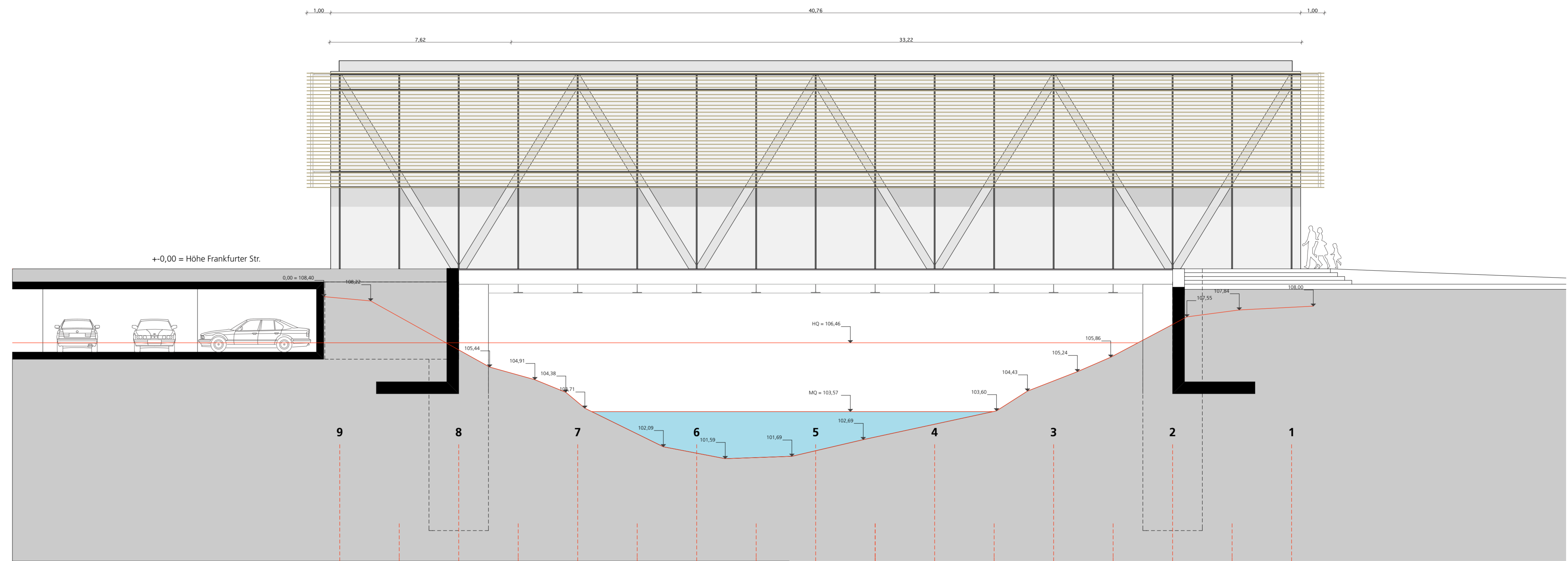
Ansicht Nordost
