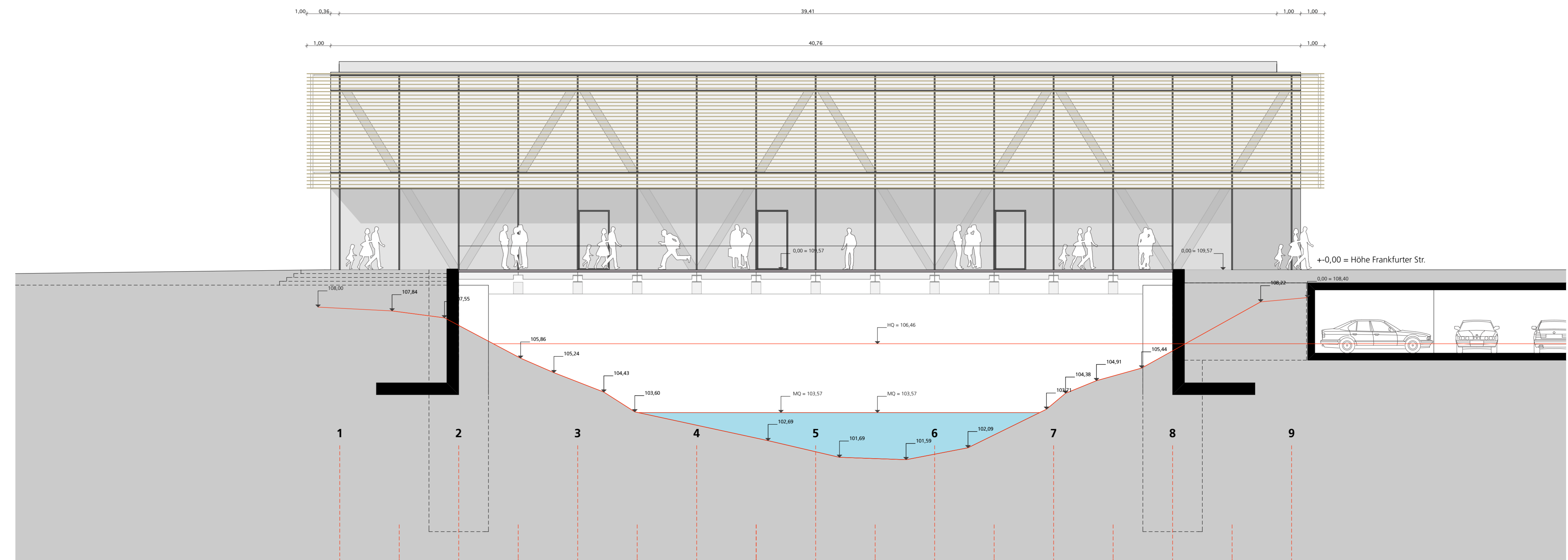
Ansicht Südwest
